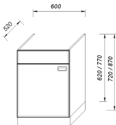
Blende – 1 Flügeltür
