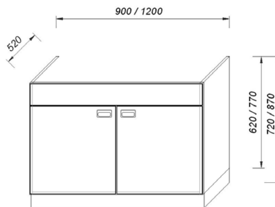
Blende – 2 Flügeltüren
